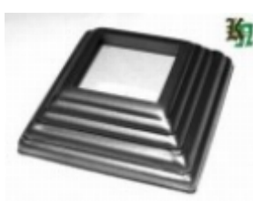
Основание блясины, арт. 13.350.01 100x100x1мм, кв.50x50мм Вес: 0.064 кг Цена: 37 руб.
