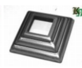
Основание баясины, арт. 13.329.01 44x44x1мм, кв.17x17мм Вес: 0.021 кг нет в наличии
